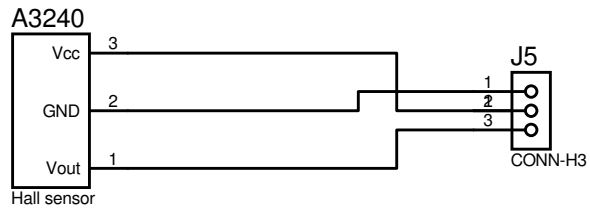
RPM-SENSOR
